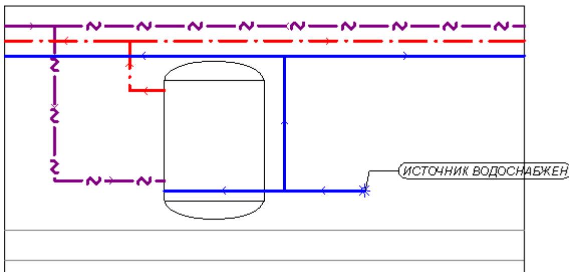
Фрагмент системы с баком - аккумулятором горячей воды
