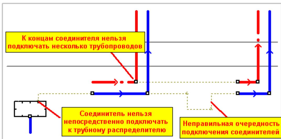
Примеры неправильного подключения соединения удаленных трубопроводов
