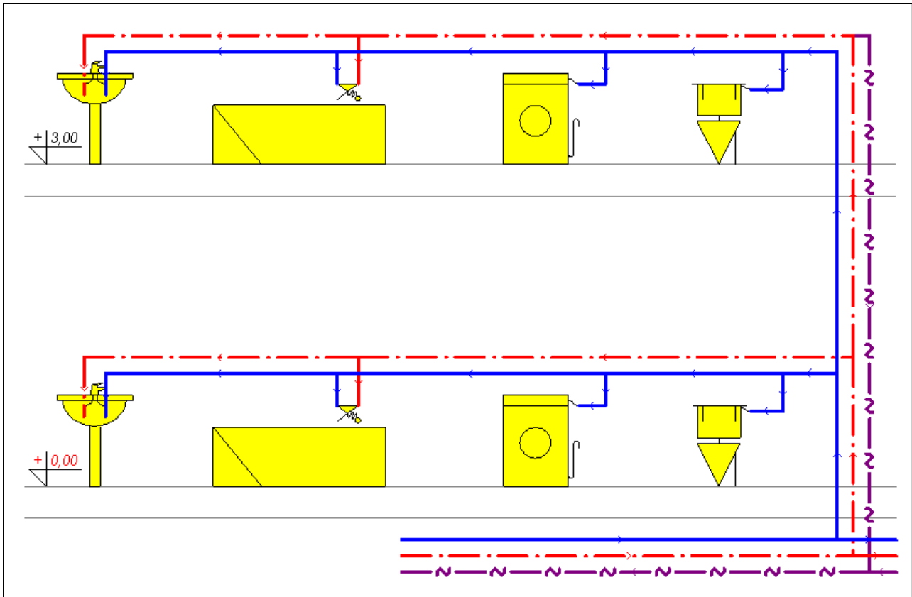
Фрагмент схемы с нарисованной сетью трубопроводов
