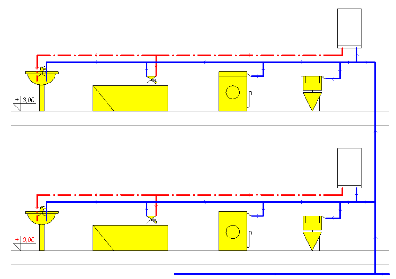
Фрагмент системы с индивидуальным водонагревателем
