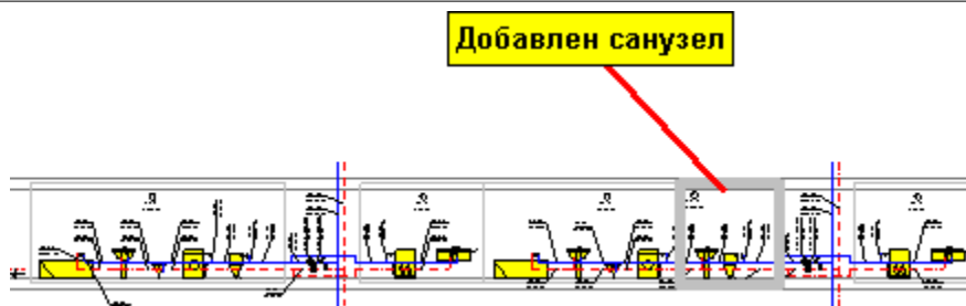
Фрагмент системы на первом этаже после добавления санузла
