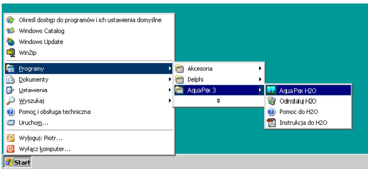
Запуск программы Aqua Pex H2O
