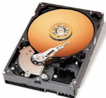
Жесткий диск (внутреннее устройство)
