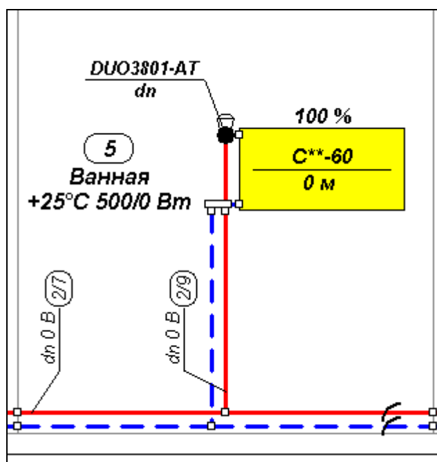
Рис. 9.17. Фрагмент рисунка с отопительным прибором, подключенным при помощи присоединительного элемента
