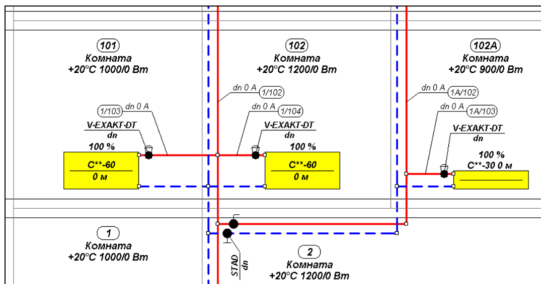
Рис. 9.19. Подсоединение стояка 1А со стояком ном. 1
