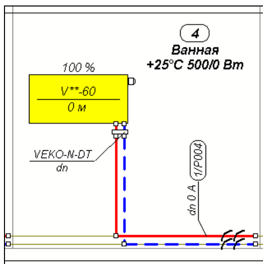
Рис. 9.22. Фрагмент рисунка с отопительным прибором тип VK
