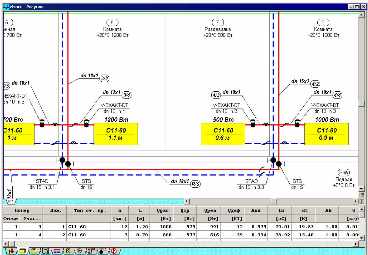
Рис. 9.14. Фрагмент схемы с итогами расчетов
