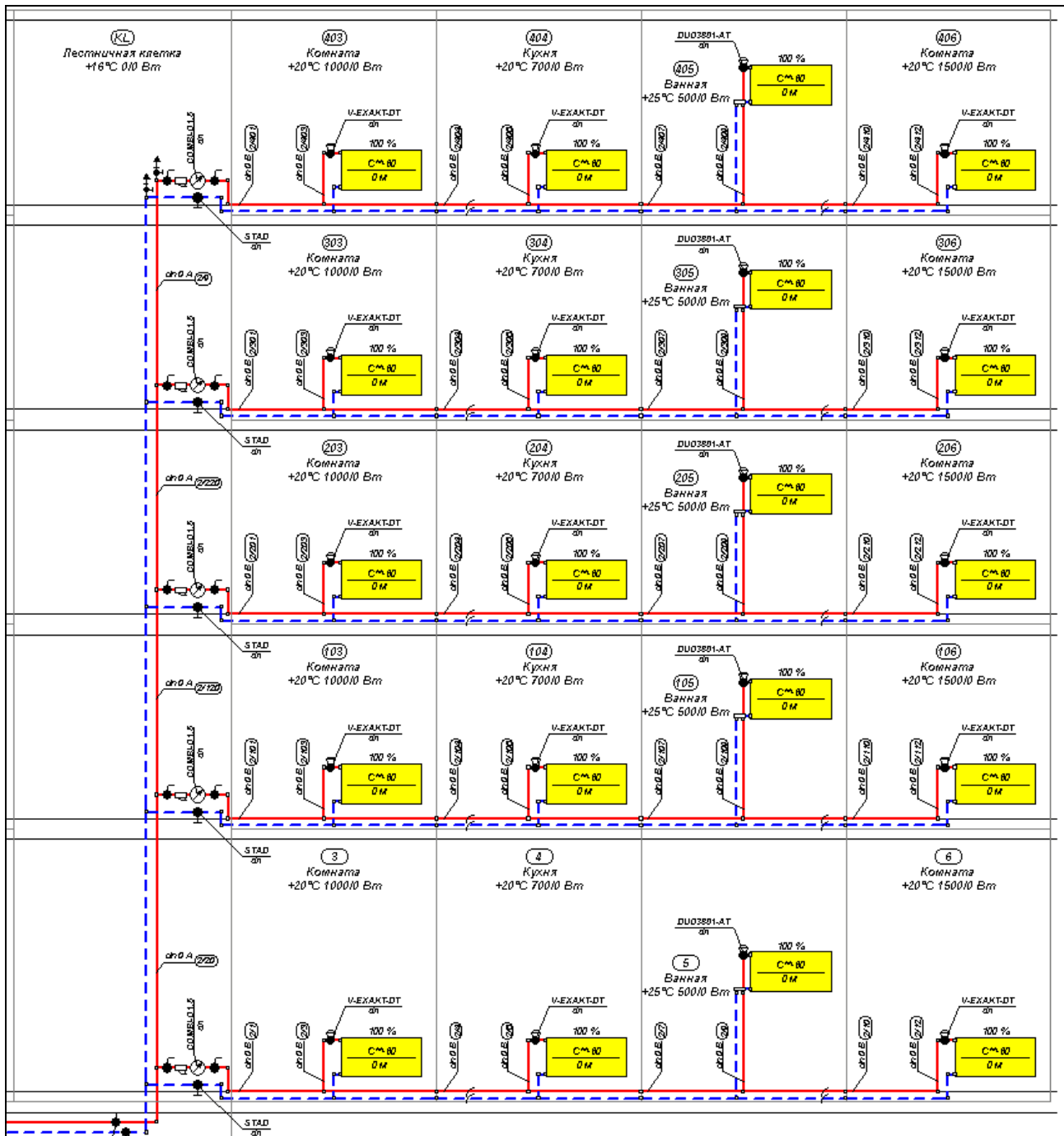
Рис. 9.18. Фрагмент схемы с поквартирной горизонтальной системой разводки
