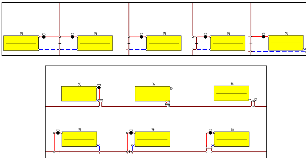
Рис. 5.62. Примеры подключения отопительных приборов в однотрубной системе
