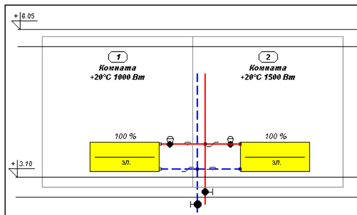
Рис. 5.27. Фрагмент с нарисованными зонами помещений
