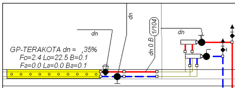
Рис. 5.54. Расположение регулирующих вентиляей рядом с подпольным отопительным прибором.
