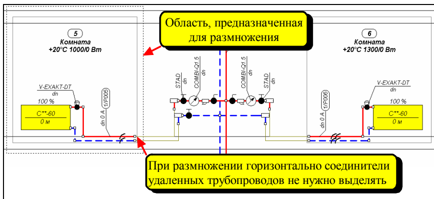
Рис. 9.21. Вставленный фрагмент распределительной системы поквартирной
