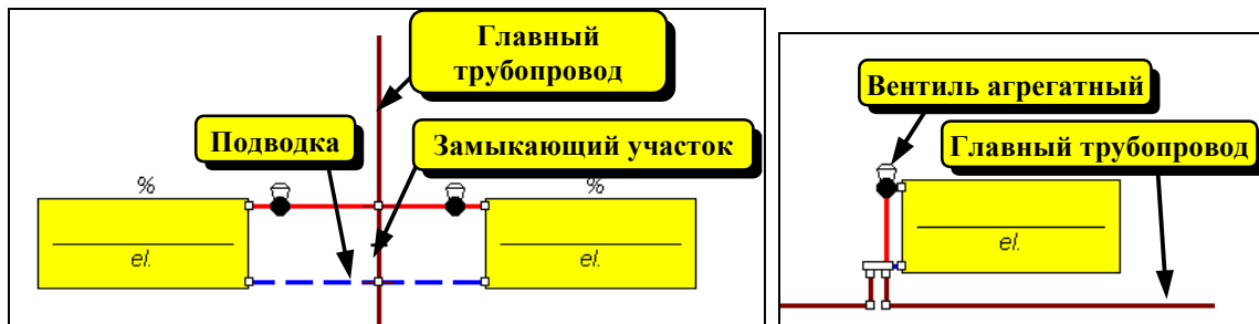
Рис. 5.61. Примеры радиаторных узлов
